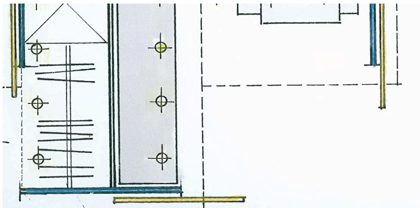
Abbildung 22: Möbelentwicklung Büro (Detailplanausschnitt) ; Zeichnung Ulrich Hollstein Innenarchitekt; Hamburg
